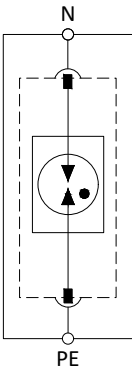
Принципиальная схема
