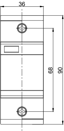
Габаритные размеры
